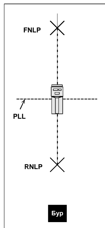
Приемник обращен в сторону от буровой установки
