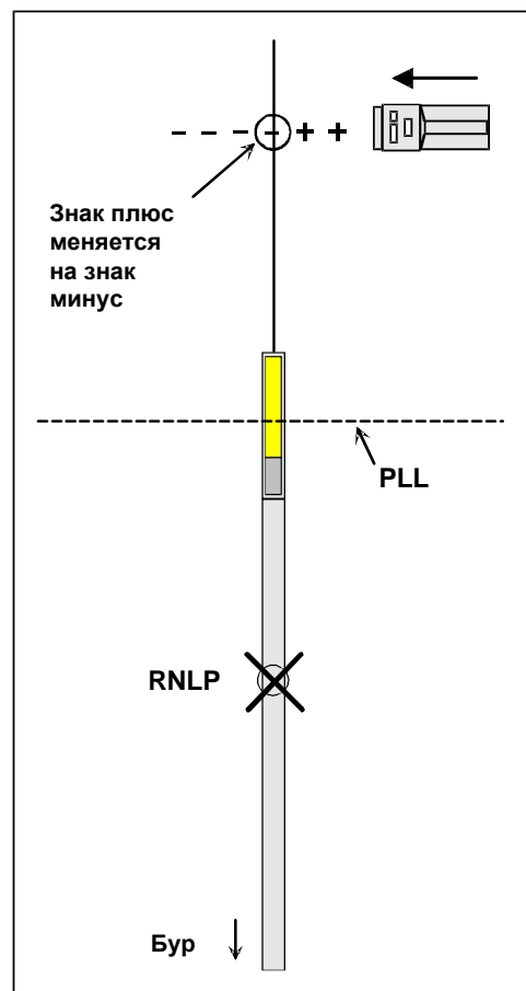
Поиск передней отрицательной точки позиционирования (FNLP) от буровой установки
