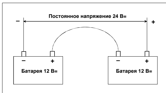
Последовательное подсоединение батарей
